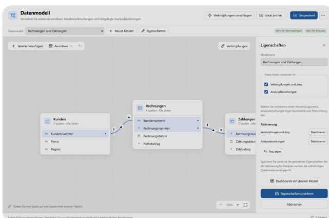
Datenmodell und Dashboard-Bibliothek in AUDIPY, Beispieldaten.
